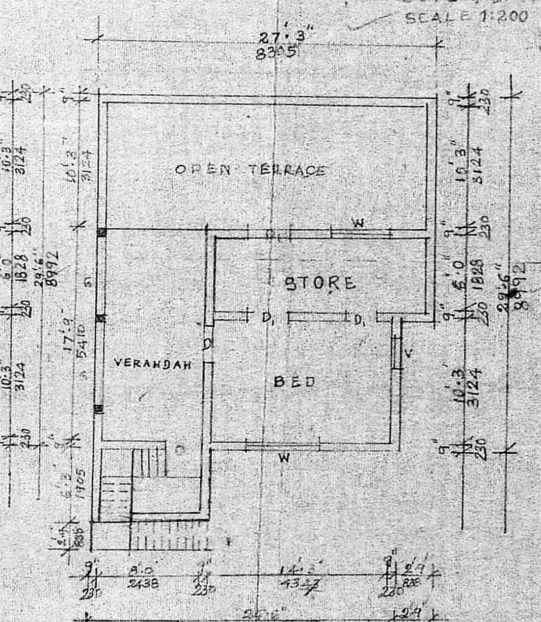
S.F. PLAN
