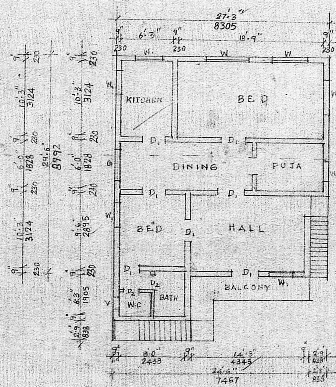
F.F. PLAN
